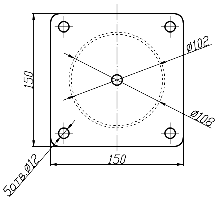
Вид А (1:2,5)
